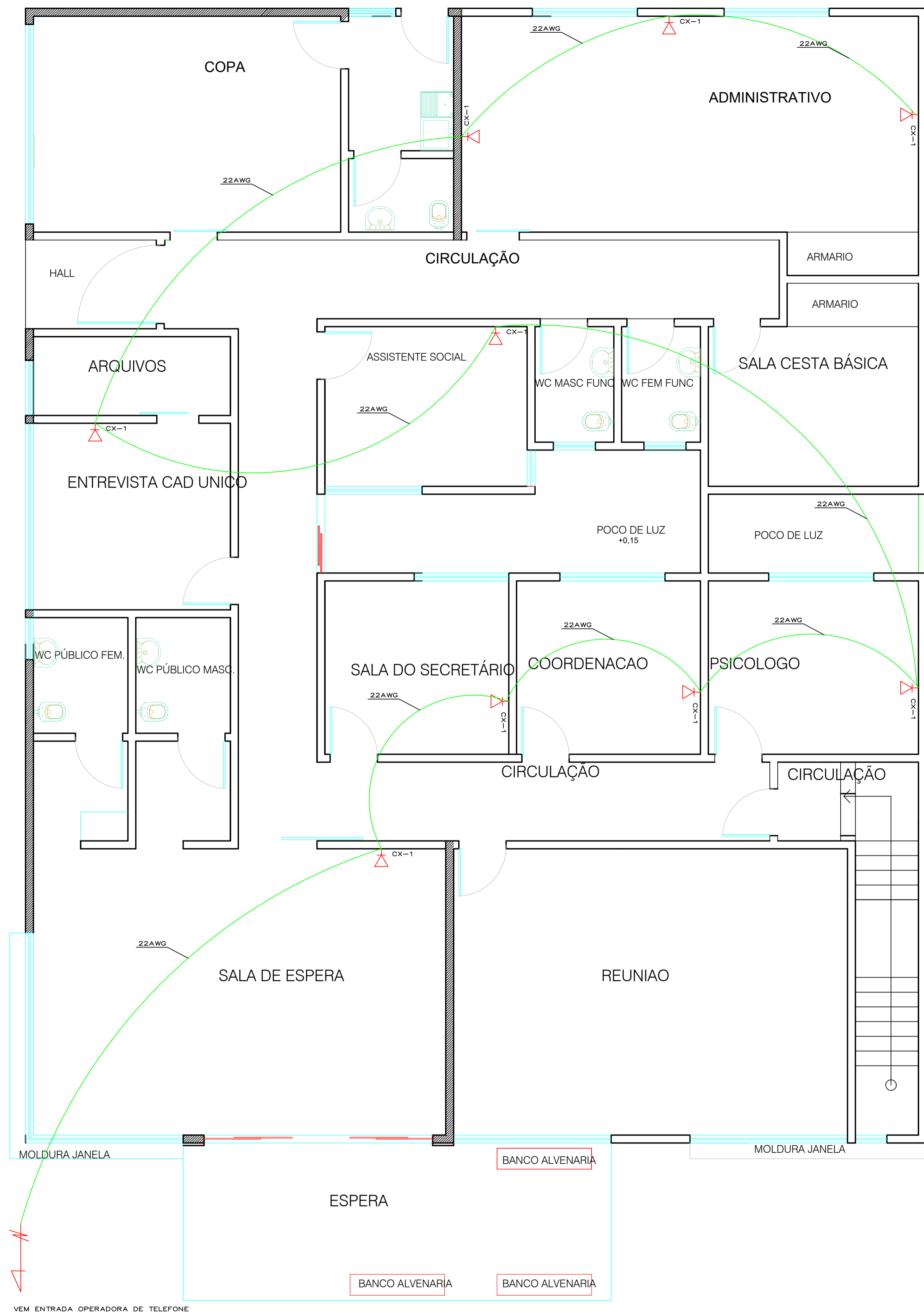
PLANTA-BAIXA NÍVEL TÉRREO
